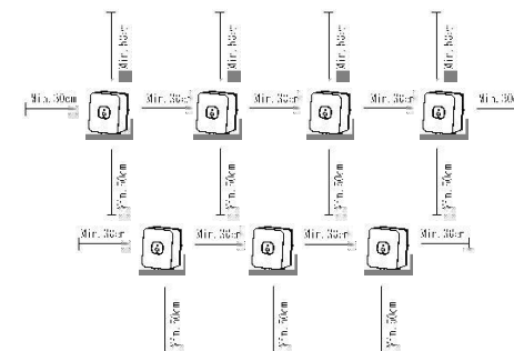
Umgebungsabmessungen von Reihenwechselrichtern
