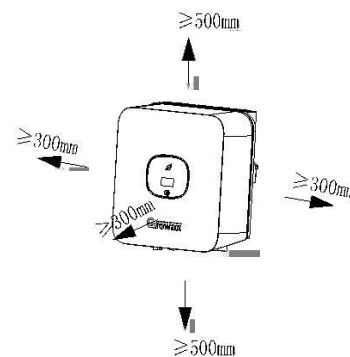
Umgebungsabmessungen eines Wechselrichters
